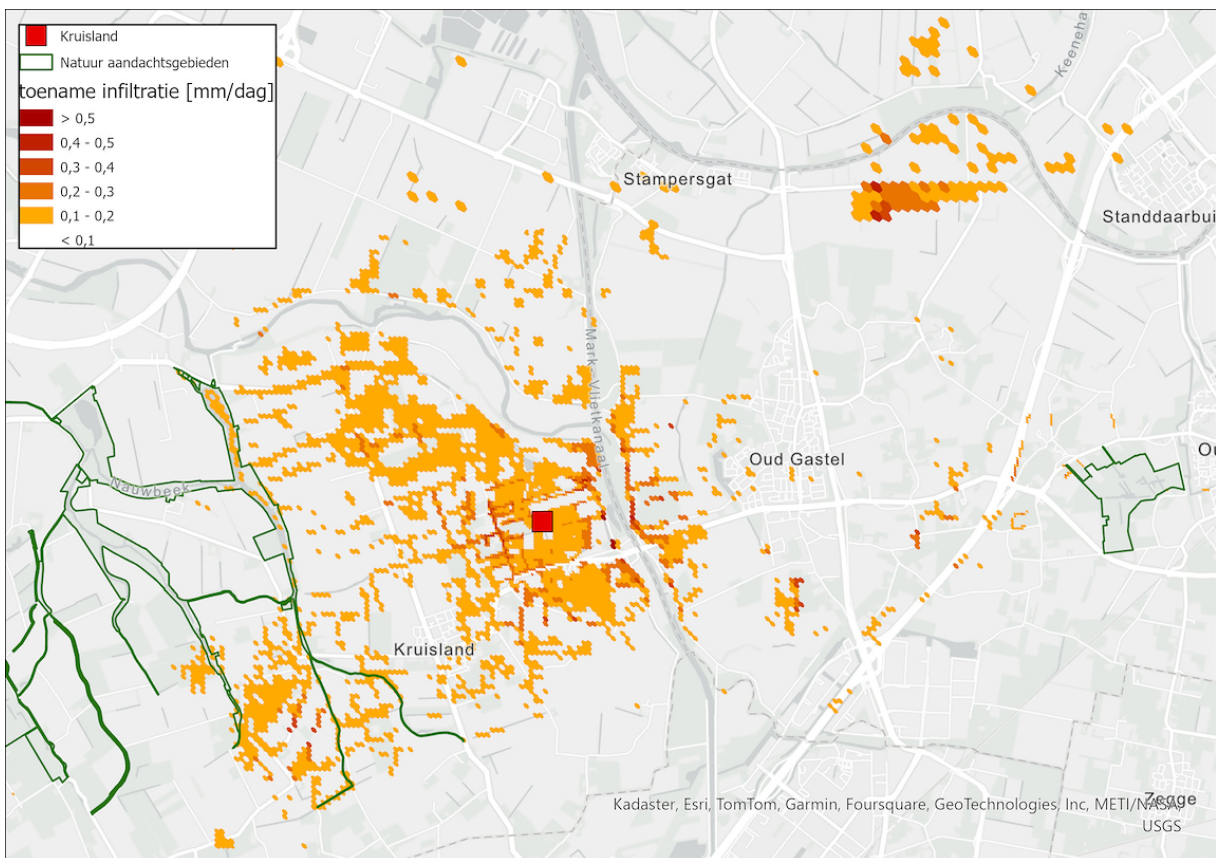
Figuur 10-7: Berekende verandering in infiltratiefluxen
