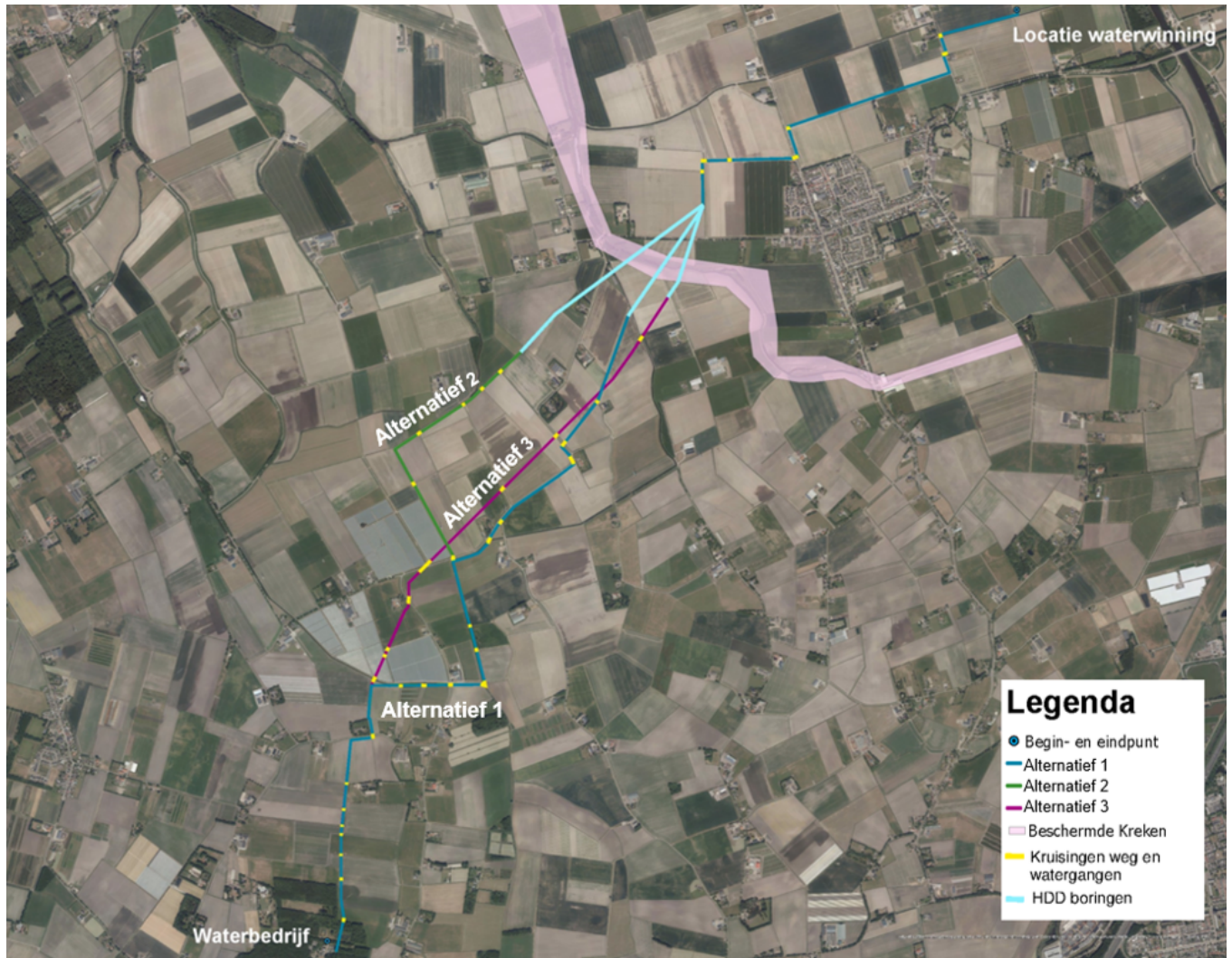
Figuur 6-1: Tracévarianten tussen de nieuwe drinkwaterwinning Kruisland en de zuivering bij het bestaande waterproductiebedrijf Wouw
