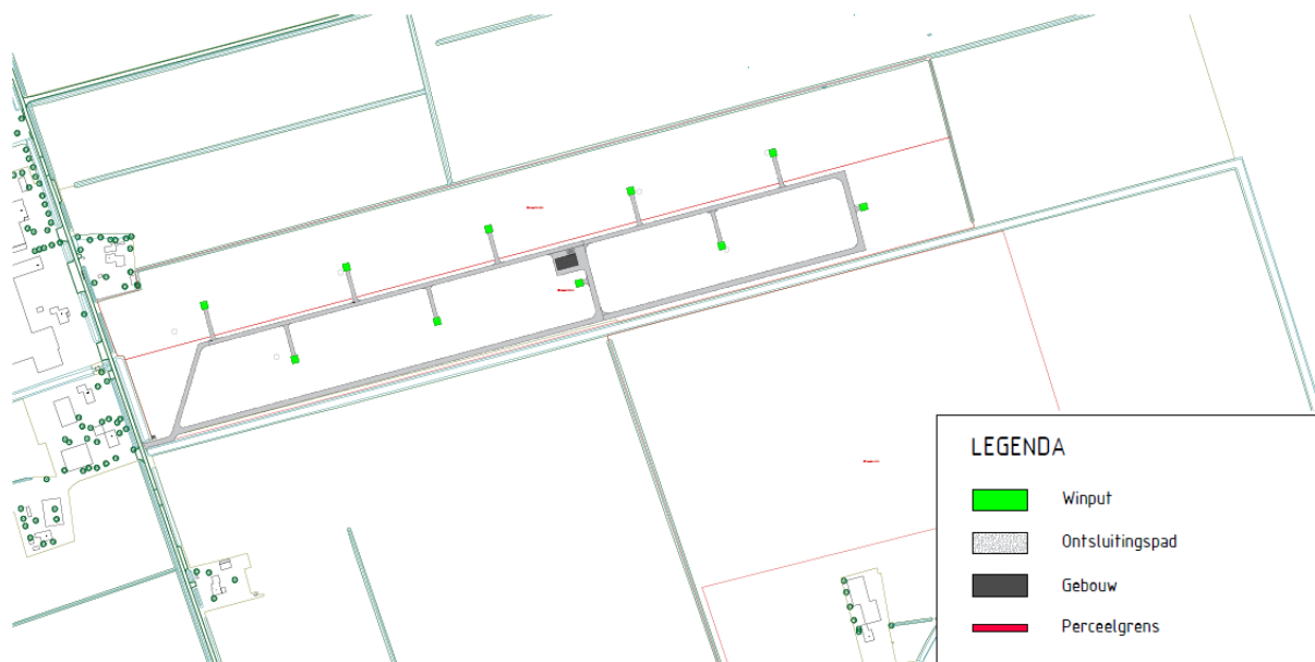
Figuur 5-1: Indicatieve indeling* van de winlocatie met tien winputten, leidingen en gebouw met daarin de installaties voor het transport, de elektriciteit en opslag. Het terrein loopt over twee percelen, beide in eigendom van Brabant Water. *Om een beeld te geven van de ligging van de winputten zijn deze indicatief ingetekend. De exacte ligging van de winputten kan mogelijk nog wijzigen.
