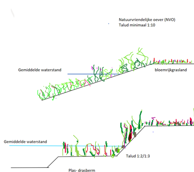
Figuur 5-3: Principe bodemprofiel natuurvriendelijke oevers
