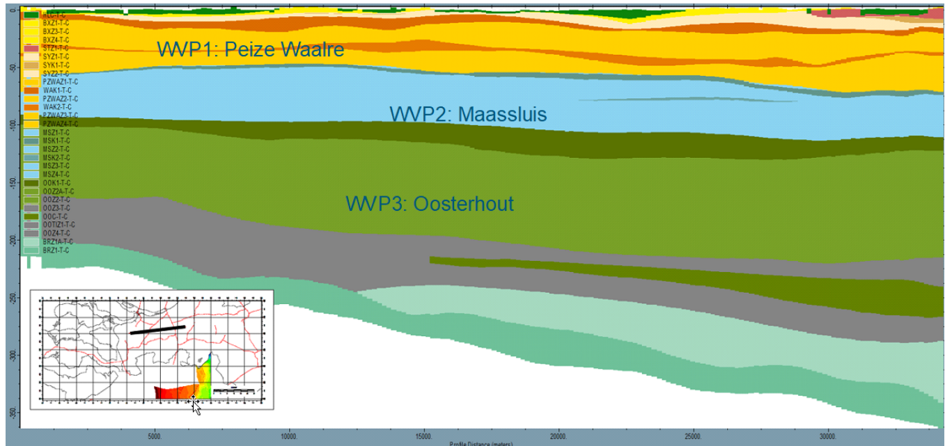
Figuur 4-3: Geohydrologisch dwarsprofiel van het zoekgebied (WVP staat voor watervoerend pakket)
