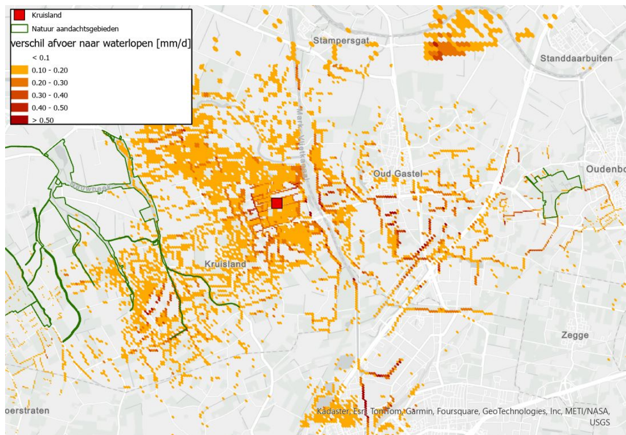
Figuur 10-8: Berekende veranderingen in de flux naar de waterlopen
