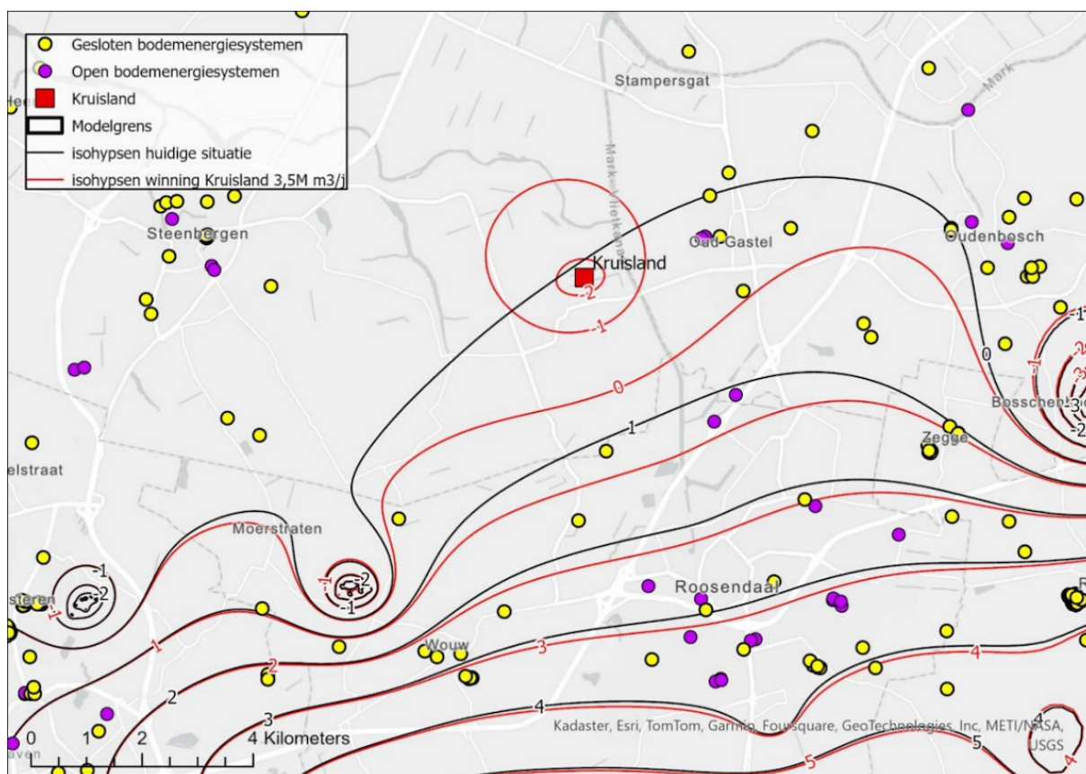
Figuur 11-11: Berekende stijghoogten in de referentiesituatie en stijghoogten na start drinkwaterwinning Kruisland ten opzichte van de ligging van bodemenergiesystemen in het watervoerende pakket van Oosterhout (bepompte pakket)
