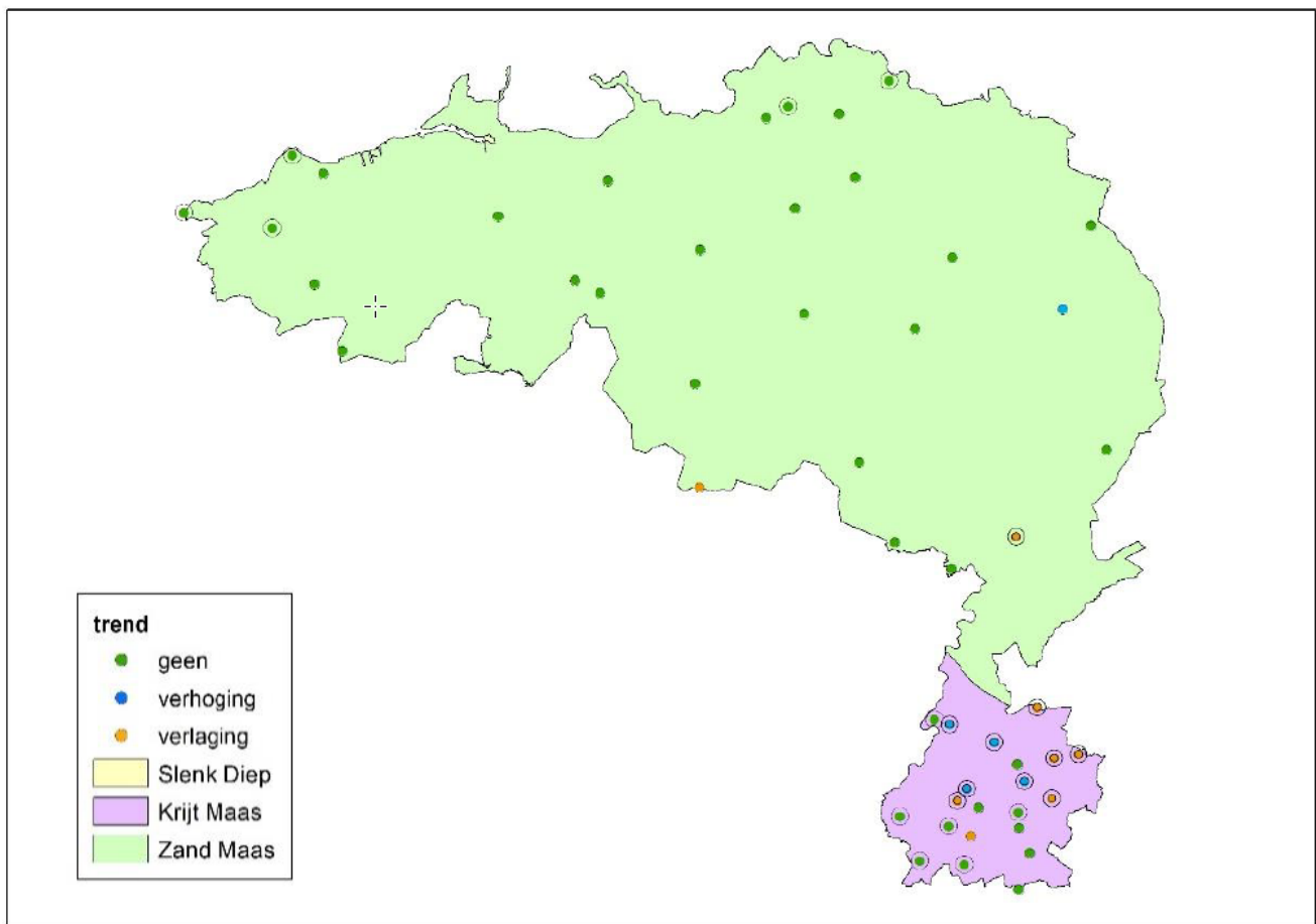
Figuur 11-4: Resultaat KRW-trendanalyse stijghoogten voor de periode 2012-2017 ten opzichte van de periode 2000-2006 in grondwaterlichamen Zand Maas en Krijt Maas. De reeksen zonder betrouwbaar tijdreeksmodel zijn omcirkeld (KWR, 2020b)
