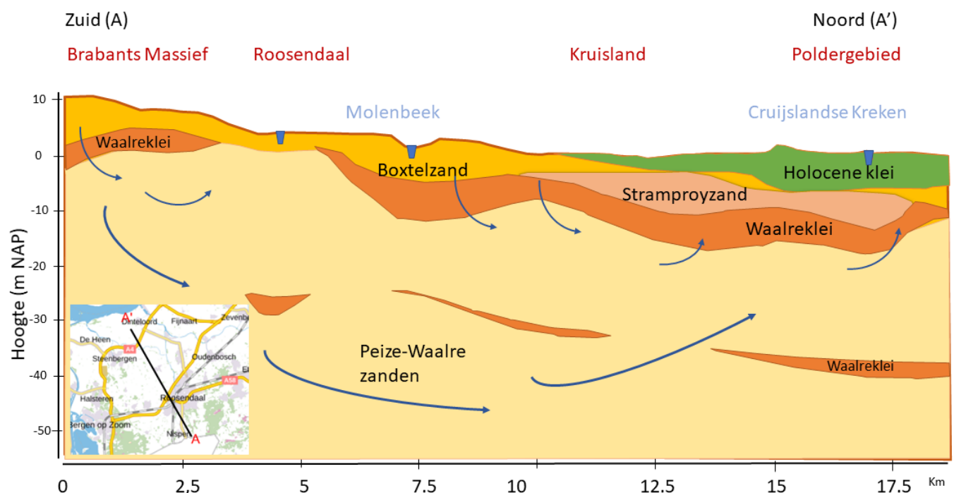
Figuur 9-1: Schematische weergave van de geohydrologie van West-Brabant met de richting van de grondwaterstroming
