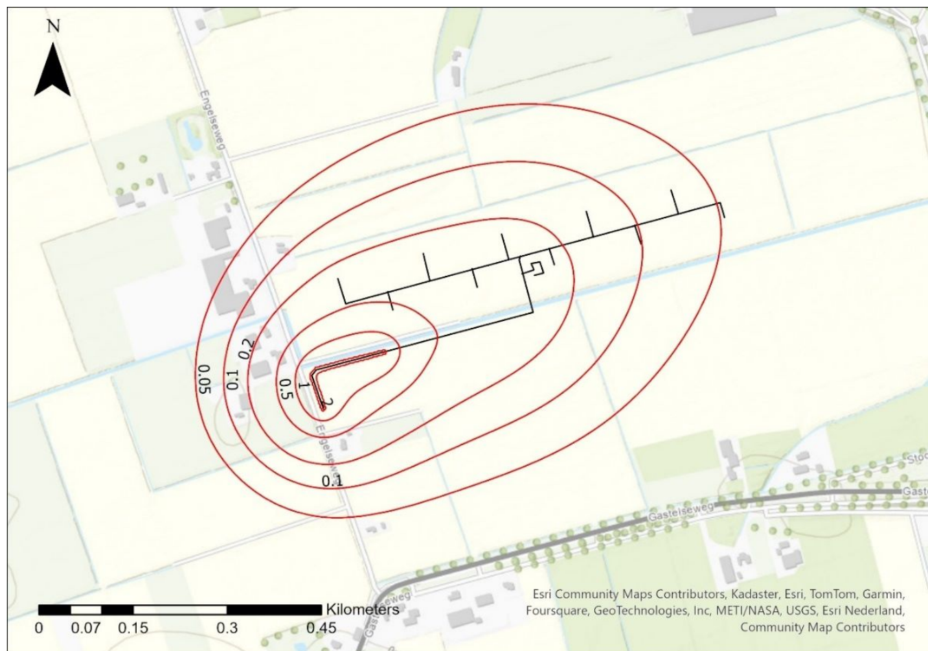
Figuur 10-16: Verlagen (in meters) in de omgeving bij GHG na aanleg laatste stuk leidingwerk (eind maand 9, indicatief en worstcase)
