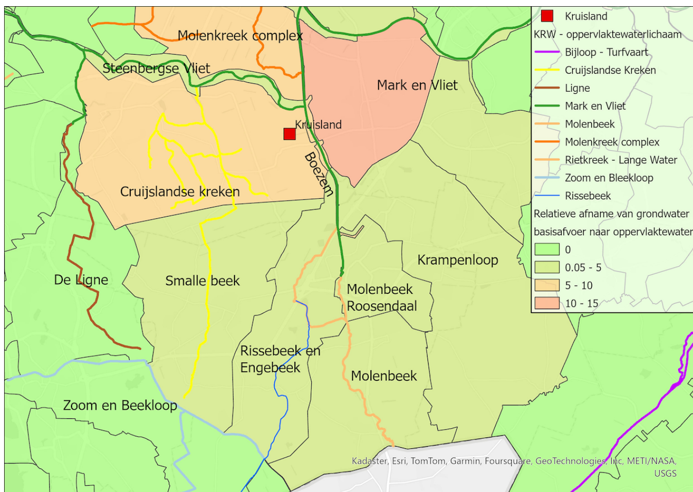
Figuur 11-9: Relatieve afname van de toestroming van grondwater naar het oppervlaktewatersysteem per deelstroomgebied (gemiddelde situatie)
