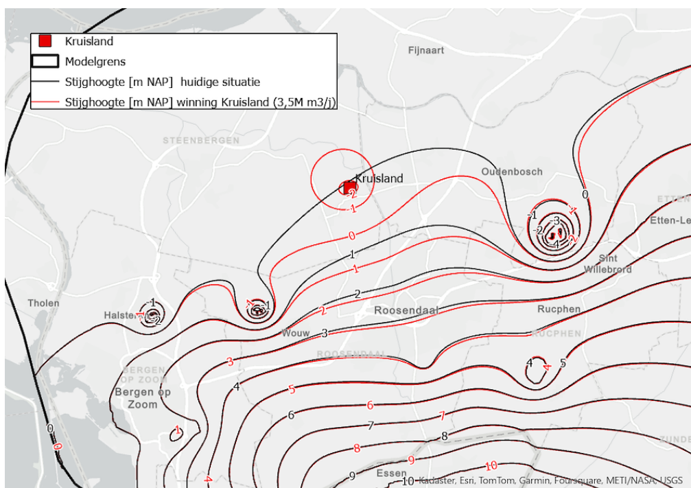
Figuur 10-10: Isohypsen in een gemiddelde situatie in het gepompte pakket (modellaag 19, Formatie van Oosterhout) (m NAP)
