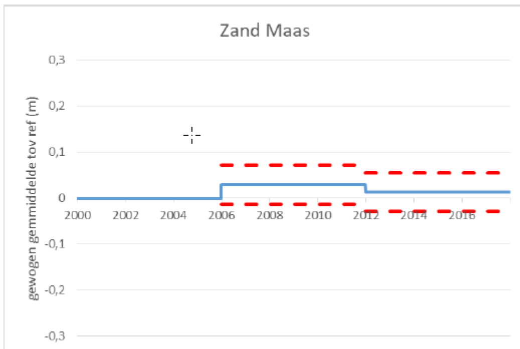
Figuur 11-5: Resultaat KRW trendanalyse Zand Maas. De y-as is het gewogen gemiddelde van de stijghoogte ten opzichte van de gemiddelde stijghoogte in de referentieperiode (2000-2005). Blauwe lijn: gemiddelde verschil t.o.v. referentieperiode. Rode gestippelde lijnen geven het 95 % betrouwbaarheidsinterval (KWR, 2020b)
