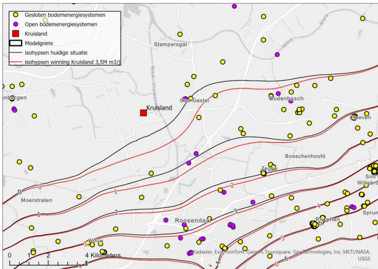
Figuur 11-10: Berekende stijghoogten in de referentiesituatie en stijghoogten na start drinkwaterwinning Kruisland ten opzichte van de ligging van bodemenergiesystemen in het watervoerende pakket van Peize-Waale
