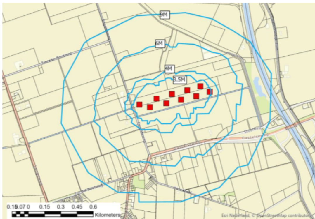
Figuur 12-1: Indicatieve berekening van de 25-jaarszones bij de variatie van wincapaciteit (in miljoen m 3 /jaar) in Kruisland
