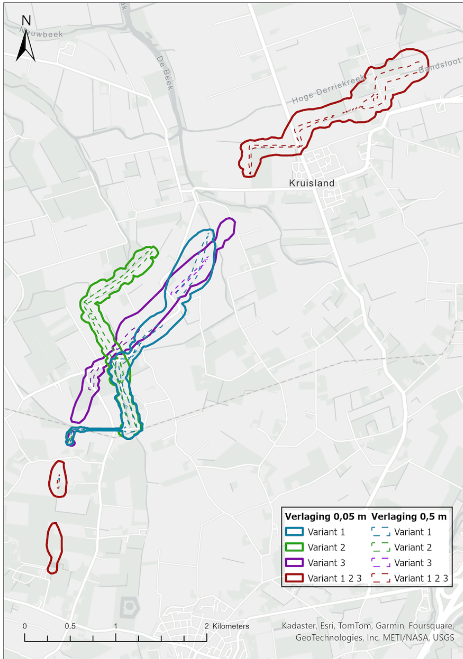
Figuur 13-1: Berekende verlagingen van de grondwaterstand als gevolg van bemaling langs de tracévarianten. Weergegeven zijn de 5 cm verlagingcontouren van de drie tracévarianten in een wintersituatie. Het begin en eindtraject van variant 1,2 en 3 zijn gelijk aan elkaar
