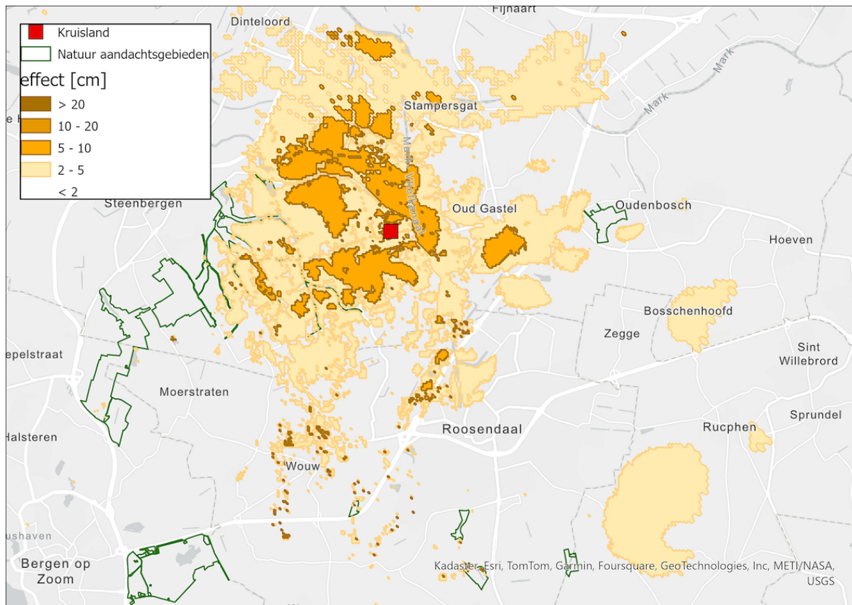
Figuur 10-4: Berekende verlaging van freatische grondwaterstand (modellaag 1) (GLG)
