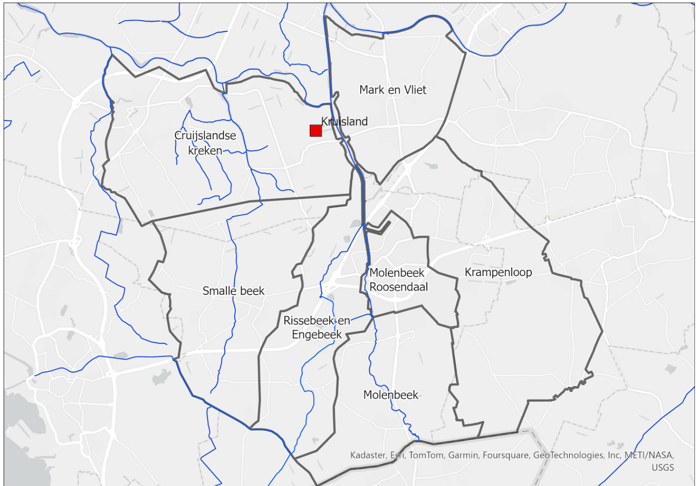
Figuur 10-13: Ligging van de acht stroomgebieden gepresenteerd in Tabel 10-2
