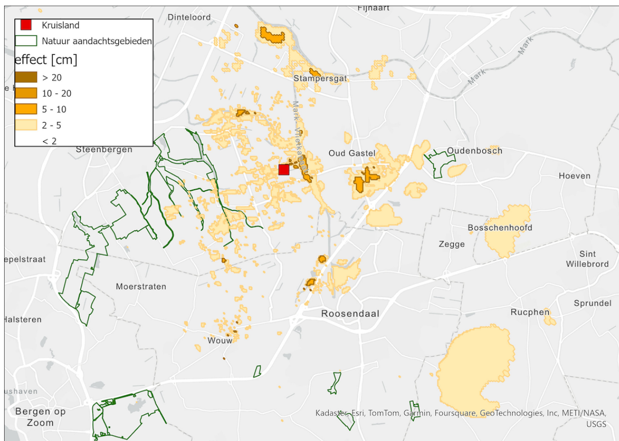
Figuur 10-3: Berekende verlaging van freatische grondwaterstand (modellaag 1) (GVG)
