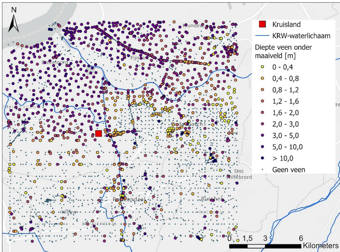
Figuur 11-12: Diepteligging van de bovenkant van de eerste veenlaag ten opzichte van maaiveld (Bron data: DINO-Loket)
