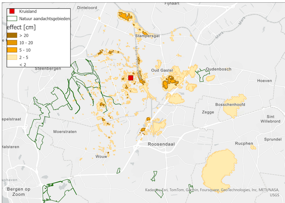
Figuur 10-2: Berekende verlaging van freatische grondwaterstand (modellaag 1) (GHG)
