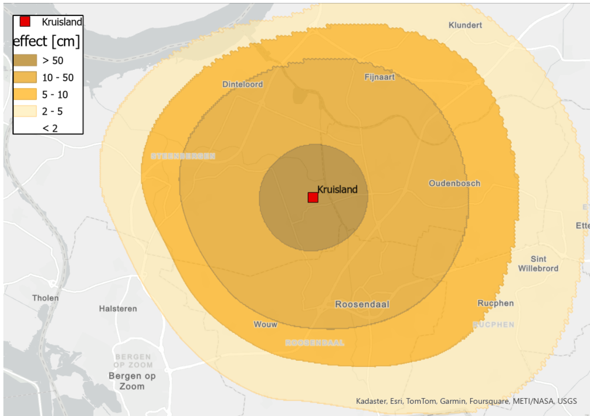
Figuur 10-1: Berekende verlaging van de stijghoogte in het bepompte pakket (Formatie van Oosterhout)
