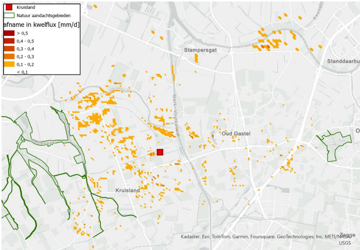
Figuur 10-6: Berekende veranderingen in kwelfluxen
