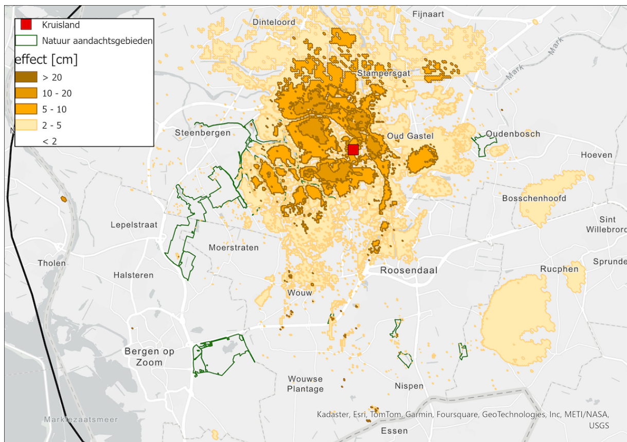
Figuur 10-5: Berekende verlaging van freatische grondwaterstand (modellaag 1) tijdens extreem droge zomer (zomer 2018)
